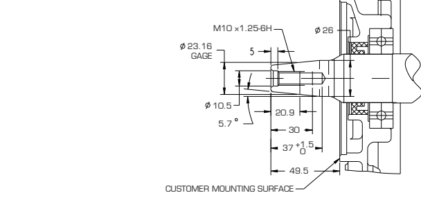
JIS 锥度轴
