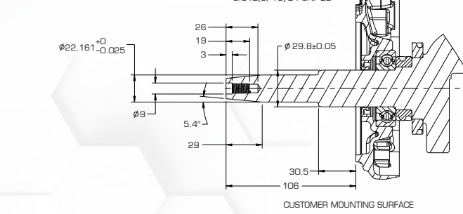
SAE 锥度轴
