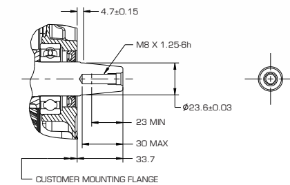
JIS 锥度轴
