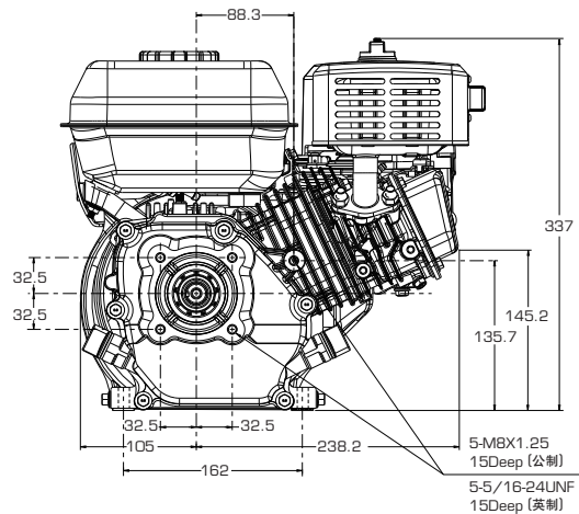
PTO
