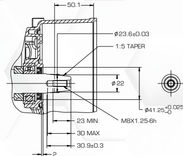
JIS锥度轴(带一体式法兰)
