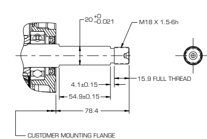
M18 螺纹轴
