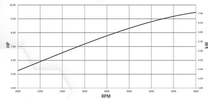
总功率曲线*
