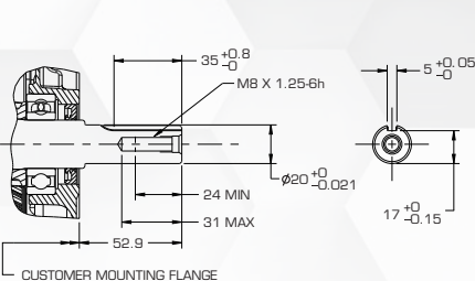
20mm 键槽轴
