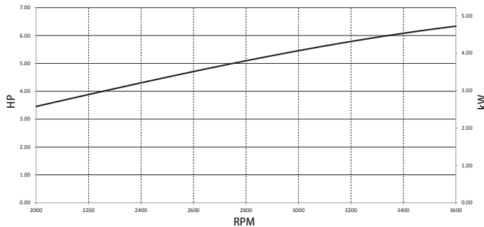
总功率曲线*
