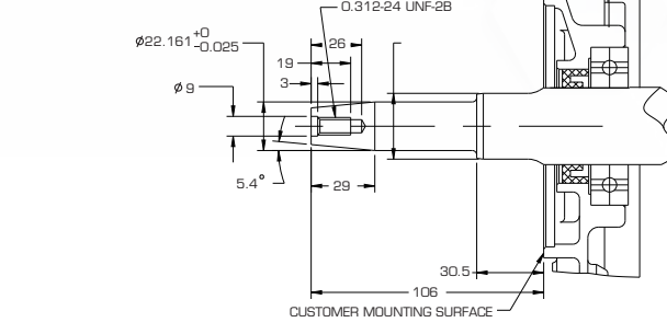
SAE 锥度轴
