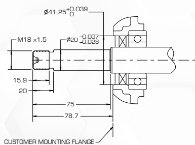
M18 x1.5 螺纹轴
