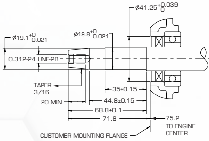
3/4" 锥度轴
