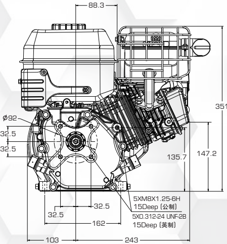
PTO
