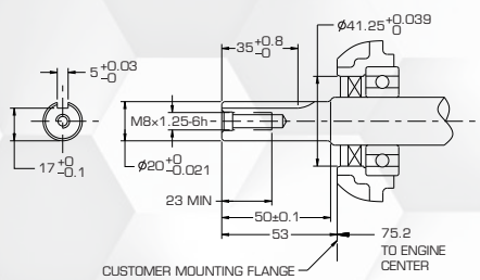
20mm 键槽轴
