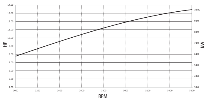
总功率曲线*
